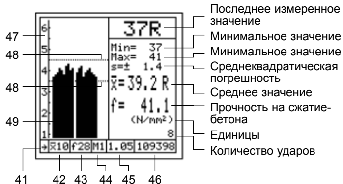
Рис. 3.1 Измерительный экран
